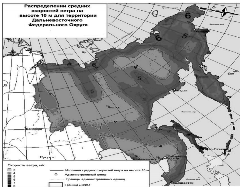
Карта распределения скорости ветра
